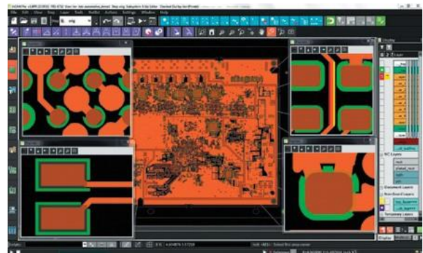
솔더 마스크 리페어(Solder Mask Repair)
